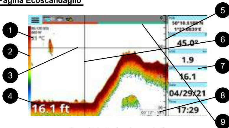
Figura 20.2 - Pagina Ecoscandaglio
