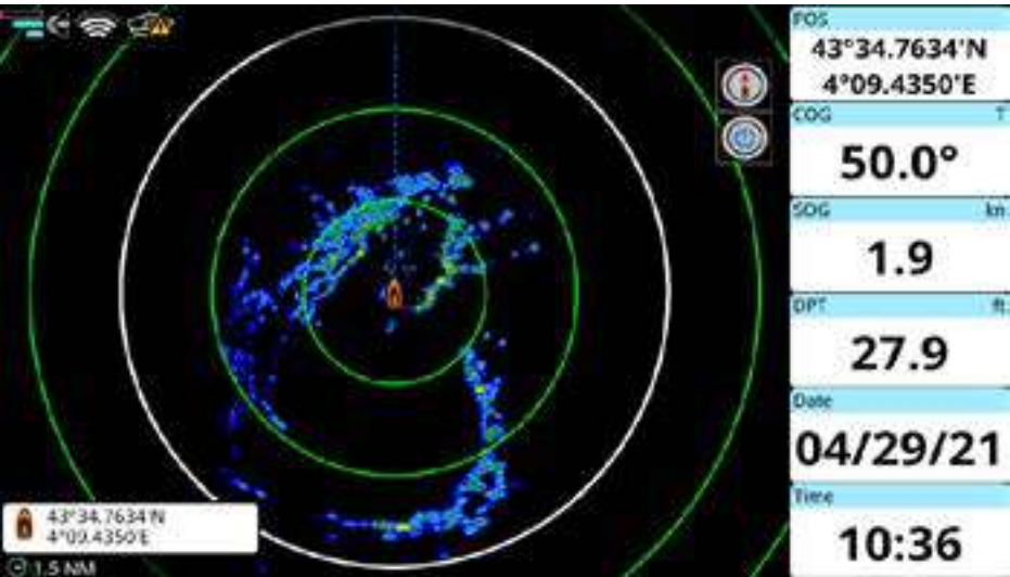
Figura 4.7 – Pagina Radar
